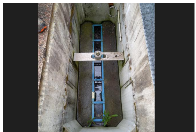
Canal de sortie avec influence aval
